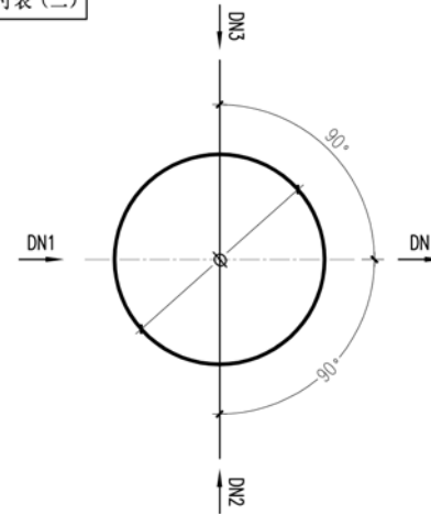
附图2: 检查井尺寸表 (二)
