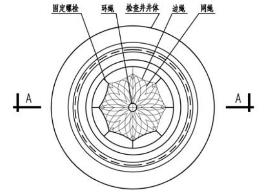
检查井筒安全网平面图1:20
