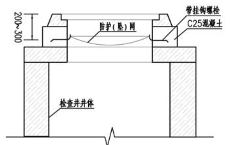
A-A剖面1:20
